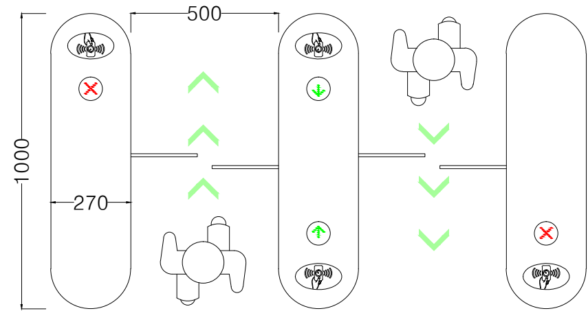
HCT 270-D TEKNİK ŞEMA
